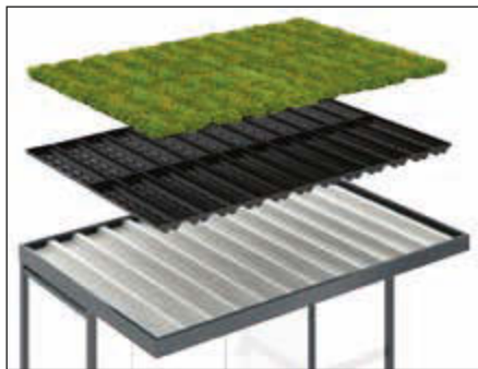
▲ Aufbauchema Dachbegrünung Wartehalle LEONIS GREEN
