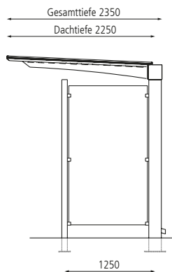
Seitenansicht
