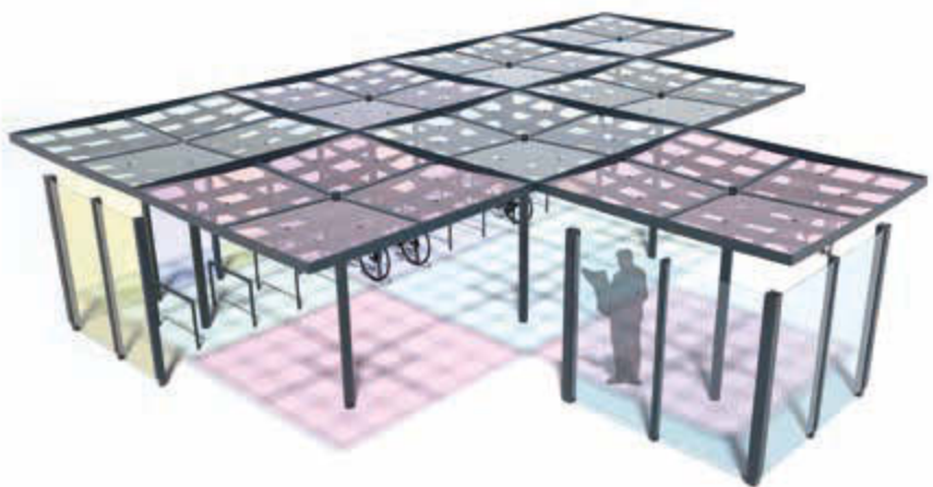
▲ Meeting-Point PIN, 8 Stück Module, Dachbreite x Dachtiefe 12300 mm x 9225 mm, auftragsbezogene Anpassung mit Seitenwänden und durchgefärbten Scheiben
