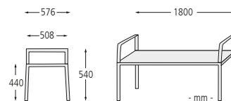
Sitzbank PREVA URBANA ohne Rückenlehne und mit Armlehnen, mit Auflage aus Edelstahl, Stahlteile in RAL 7016 anthrazitgrau
