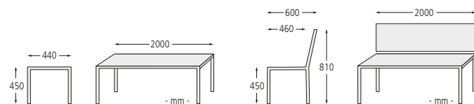
▲ Sitzbank MANTUA mit Rückenlehne, Aluminium in Durmast Eichenholzoptik-Effekt, Stahlteile in RAL 9005 tiefschwarz
