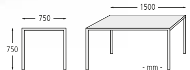
▲ Tisch CIMA mit Holzaufgabe, in RAL 7016 anthrazitgrau
