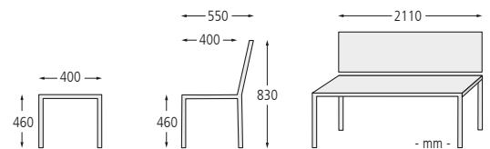
▲ Sitzbank NATURA ohne Rückenlehne, mit Escheholzbelattung, Stahlteile in RAL 7016 anthrazitgrau
