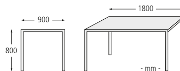
Bank-Tisch-Kombination RIMINI bestehend aus Sitzbank mit und ohne Rückenlehne und einem Tisch, in RAL 3004 purpurrot
