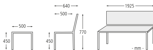
Sitzbank TAURUS mit Rückenlehne, Stahlteile in RAL 7016 anthrazitgrau
