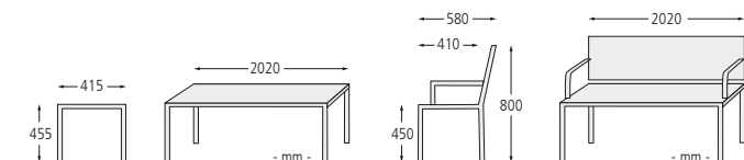
Sitzbank INTAL mit Rückenlehne, Stahlteile in RAL 9007 graualuminium, Beton beschichtet in grau
