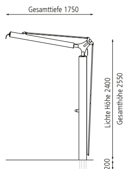
Seitenansicht
