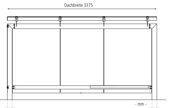
Frontansicht
