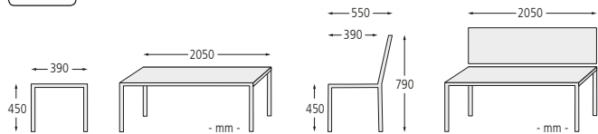
► Sitzbank BRNO ohne Rückenlehne, Stahlteile in RAL 7021 schwarzgrau
