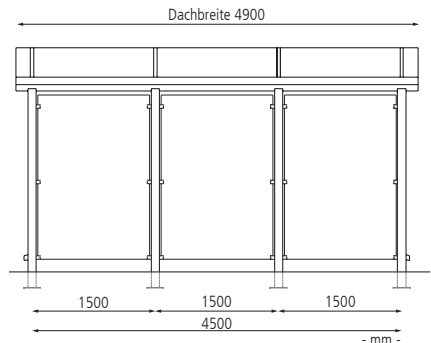
Frontansicht
