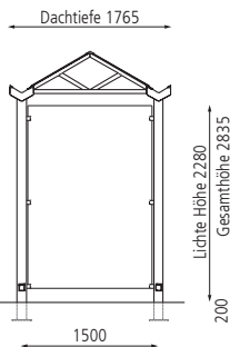
Seitenansicht
