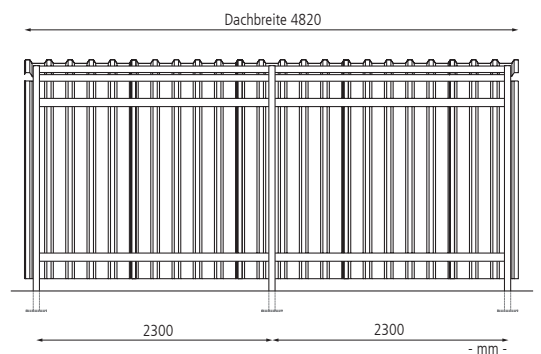
Frontansicht
