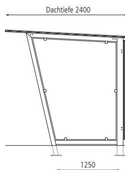
Seitenansicht
