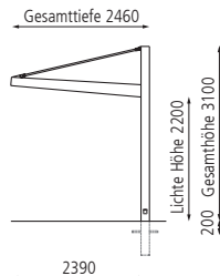
Seitenansicht, einseitig
