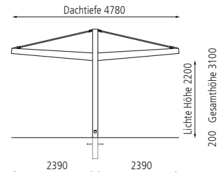
Seitenansicht, doppelseitig
