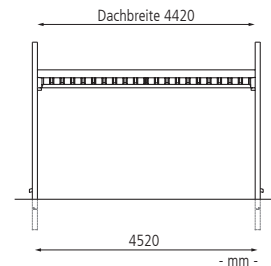
Frontansicht
