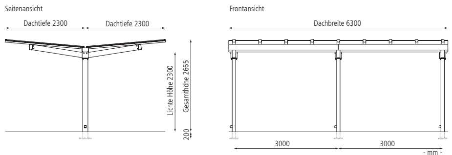
Fahrradüberdachung TUCANA, Dachbreite x Dachtiefe 6300 mm x 4600 mm, Rück- und Seitenwände ESG, Klarglas, Sitzbank RIMINI, Fahrradanhänger FLINT, Servicestation ASSIST PREMIUM, Abfallbehälter CIMA, Stahlkonstruktion in RAL 7016 anthrazitgrau
