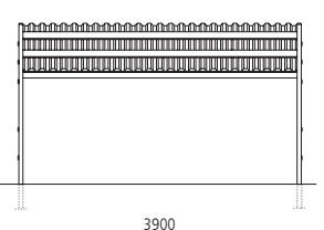
Frontansicht
