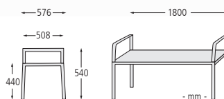
▲ Sitzbank PREVA URBANA ohne R ckenlehne und mit Armlehnen, Stahlteile in RAL 7016 anthrazitgrau
