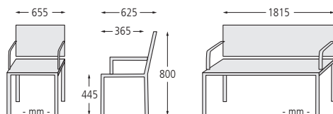
► Sitz EMAU mit Rückenlehne, mit Jatobaholzbelattung
