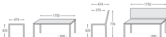
Sitzbank FOLA mit Rückenlehne, Stahlteile in eisenglimmergrau
