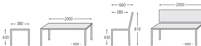
Bank-Tisch-Kombination VENEDIG, mit Escheholzbelattung, bestehend aus einem Tisch und Sitzbank ohne und mit Rückenlehne
