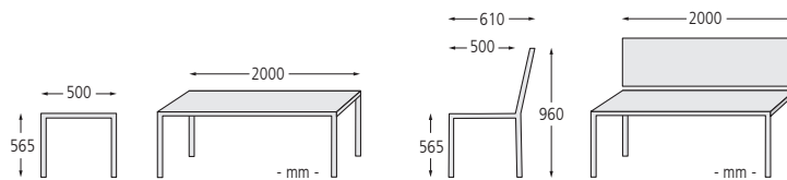
▲ Sitzbank ANDROMEDA WOOD mit Rückenlehne, mit Kiefernholzbelattung, Beton in natur
