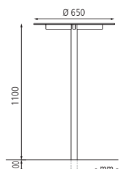
Stehtisch BISTROT mit HPL-Auflage in Black 0080, Stahlteile in DB 703 eisenglimmer
