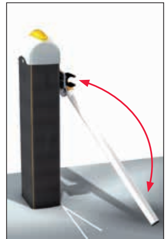
▲ Kollisionskupplung BASIC beim Auffahren auf den Schrankenbaum rastet dieser aus seiner Halterung aus und fällt nach unten
