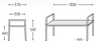
▲ Sitzbank PREVA URBANA ohne Rückenlehne und mit Armlehnen, Stahlteile in RAL 7016 anthrazitgrau
