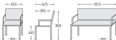
► Sitz EMAU mit Rückenlehne, mit Jatobaholzbelattung
