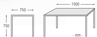
▲ Tisch CIMA mit Holzauflage, Stahlteile in RAL 7016 anthrazitgrau
