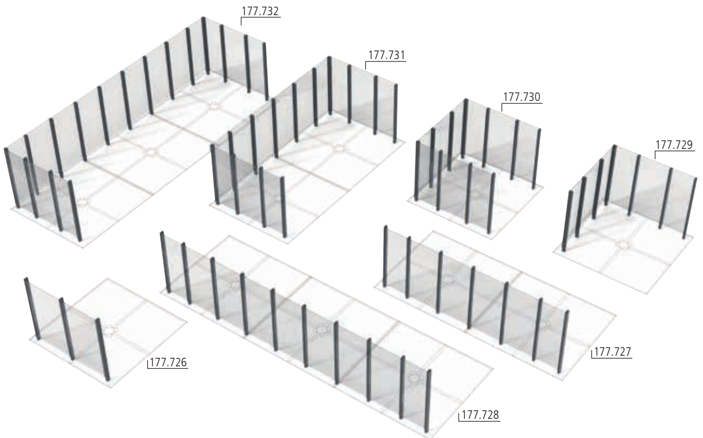
Windschutzwand PIN SCREEN, mit Einscheibensicherheitsglas, Klarglas mit Siebdruckstreifen, Meeting-Point PIN, Sitzbank NATURA, Pflanzbehälter MALOUT, Stahlkonstruktion in RAL 7046 telegrau
