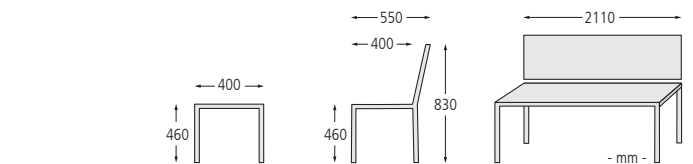
▲ Sitzbank NATURA ohne Rückenlehne, mit Escheholzbelattung, Stahlteile in RAL 7016 anthrazitgrau
