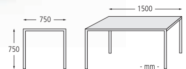
▲ Tisch CIMA mit Holzauflage, Stahlteile in RAL 7016 anthrazitgrau
