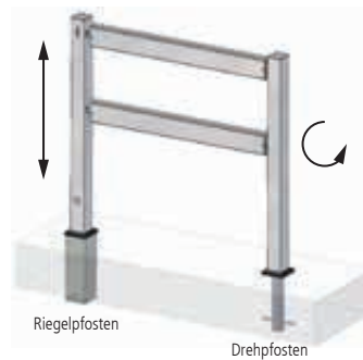
Gattersperre PERKO - schwenkbar, aus Aluminium, weiß pulverbeschichtet mit roten Reflexstreifen, Sperrbreite 1,0 m
