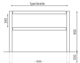
Gattersperre PERKO - schwenkbar, aus Aluminium, weiß pulverbeschichtet mit roten Reflexstreifen, Sperrbreite 1,0 m
