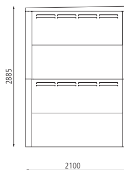
Seitenansicht
