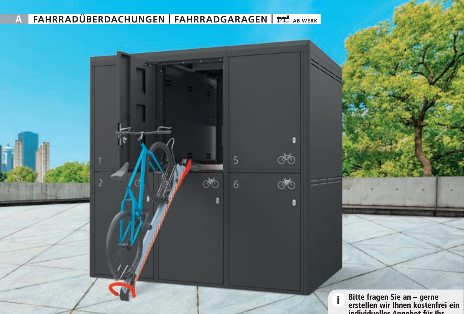
Fahrradgarage FULLERTON-KEY XL für 6 Fahrräder, zweistöckig, Höhe x Breite x Tiefe 2885 mm x 2912 mm x 2100 mm, Stahlkonstruktion in RAL 7016 anthrazitgrau
