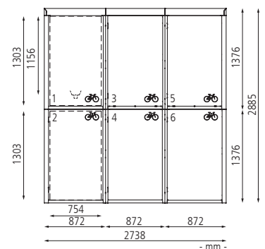
Frontansicht
