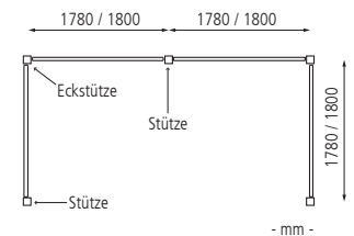
▲ Fenstermodul aus Edelstahl für WPC-Wandelement
