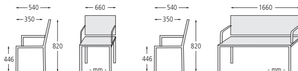
Sitz und Sitzbank BASIC, Stahlteile in RAL 7016 anthrazitgrau
