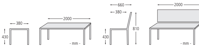
Sitzbänke VENEDIG ohne und mit Rückenlehne und Tisch VENEDIG, mit Eschenholzbelattung
