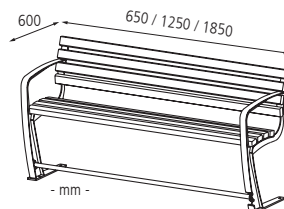
Sitzbank SENIOR, 2-Sitzer mit Armlehnen
