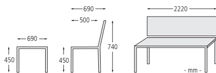
▲ Sitzbank TAURUS ohne Rückenlehne, Stahlteile in RAL 7016 anthrazitgrau
