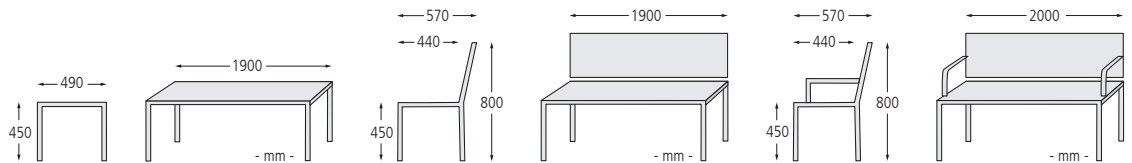
◀ Sitzbank FJORDPARK ohne Rückenlehne, Stahlteile in RAL 7016 anthrazitgrau
