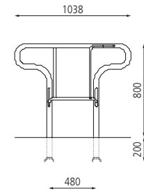
▲ Radeinstellung doppelseitig hoch, zum Aufdübeln bei -200 mm, kurzer Bügel, (Reihenaufstellung)
