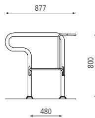
▲ Radeinstellung einseitig hoch, zum Aufdübeln, kurzer Bügel, (Reihenaufstellung)
