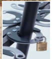
▲ Detail: Lenkersicherung
