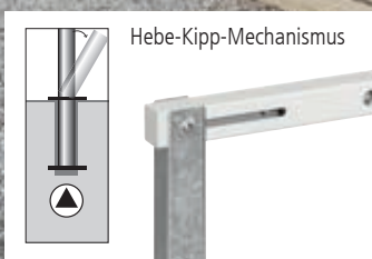
Sperrpfosten GERNIKA NEW zum Aufdübeln, einseitig kippbar, mit Bodenplatte, mit Profilzylinderschloss, in RAL 9010 reinweiß mit roten Reflexstreifen
