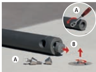
A - Spannegelsatz im Poller lösen und herausnehmen. B - gebrochene Verbindungsstücke aus Poller und Bodenhülse entnehmen.
