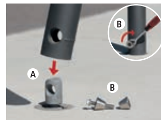
A - Poller auf Verbindungsstück setzen. B - Spannegelsatz einsetzen und festziehen.
