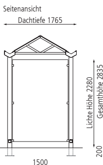
Wartehalle WAAGE, Dachbreite x Dachtiefe 6400 mm x 1765 mm, Rück- / Seitenwände ESG, Klarglas, mit Siebdruckdekor Raute, Drahtgittersitzbank TARVIS, Stahlkonstruktion in RAL 6024 verkehrsgrün
