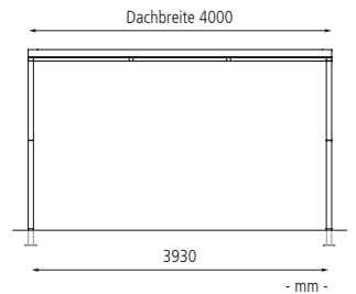
Frontansicht
