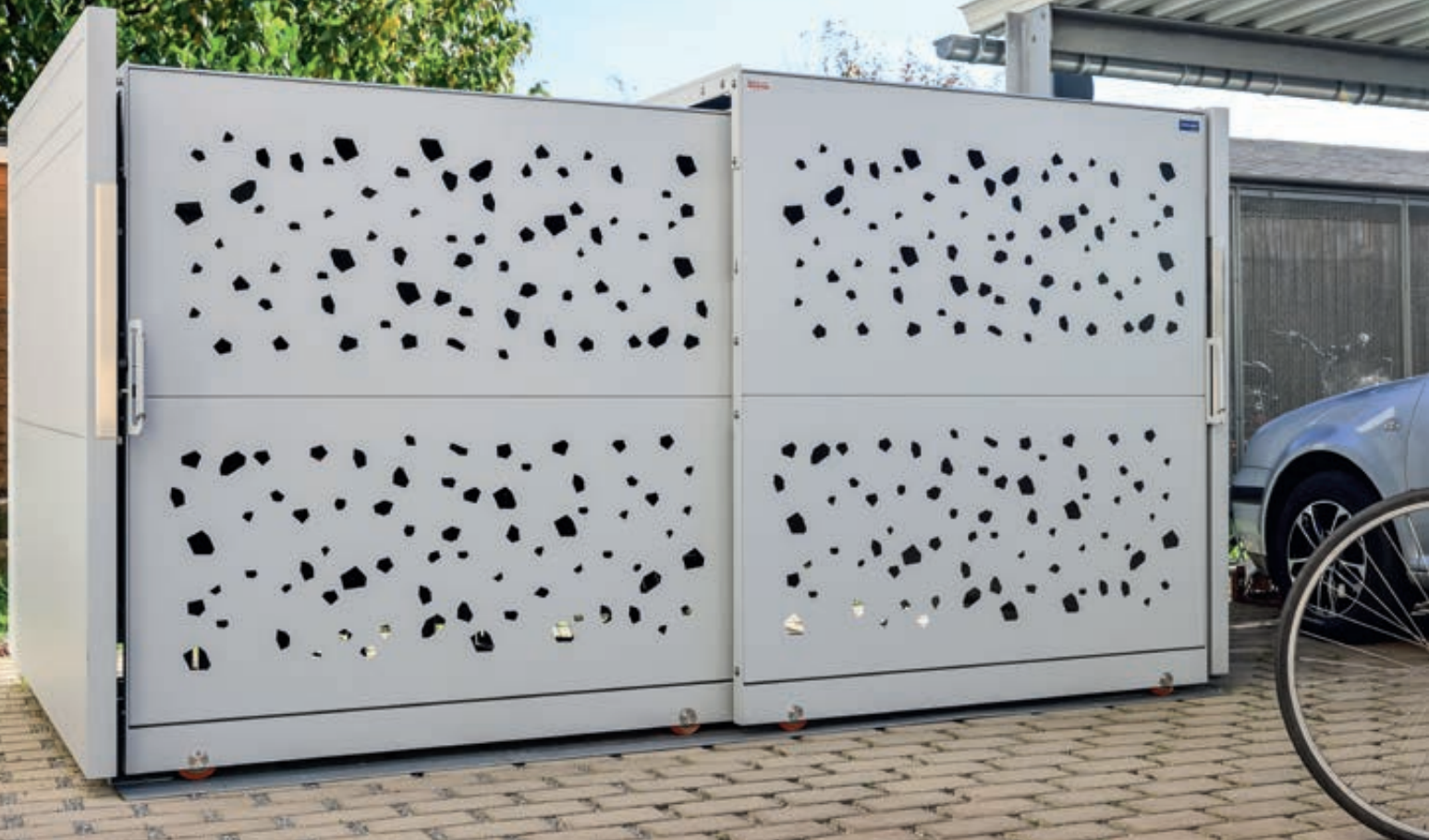
Fahrradgarage STYLEOUT® BIKE TOMO, Rück-, Seitenwände und Schiebetüren in RAL 9006 weißaluminium, Dach Aluminium eloxiert
