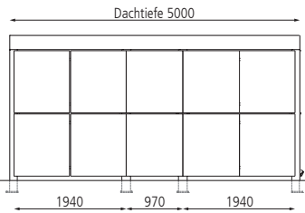
Seitenansicht für 6 Stück 4-Rad-Abfallgroßbehälter
