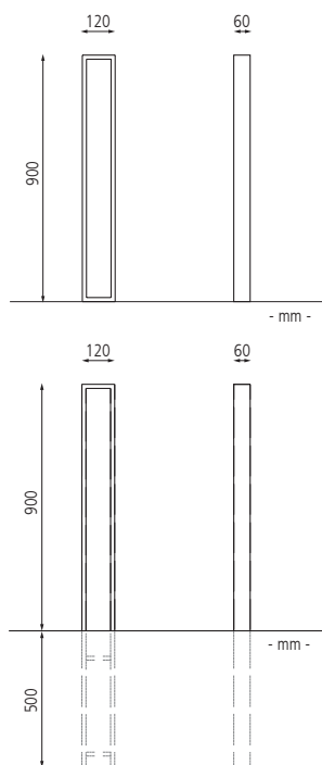
◀ Anlehnbügel LOWELL, zum Aufdübeln, in Cortenstahl
