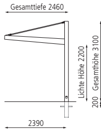
Seitenansicht, einseitig
