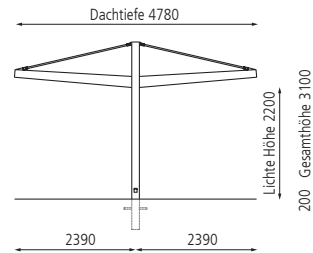
Seitenansicht, doppelseitig
