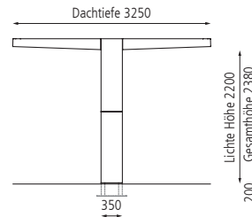
Seitenansicht, doppelseitig
