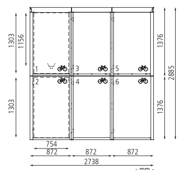
Frontansicht
