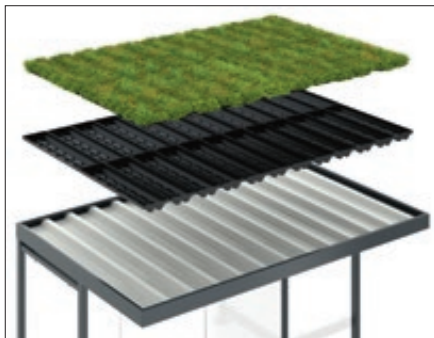
▲ Aufbauschema Dachbegrünung Raucherunterstand AQUILA GREEN
