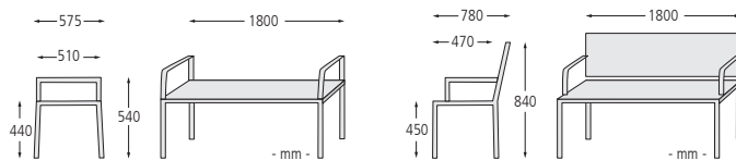
▲ Sitzbank PREVA URBANA ohne Rückenlehne und mit Armlehnen, Stahlteile in RAL 7016 anthrazitgrau
