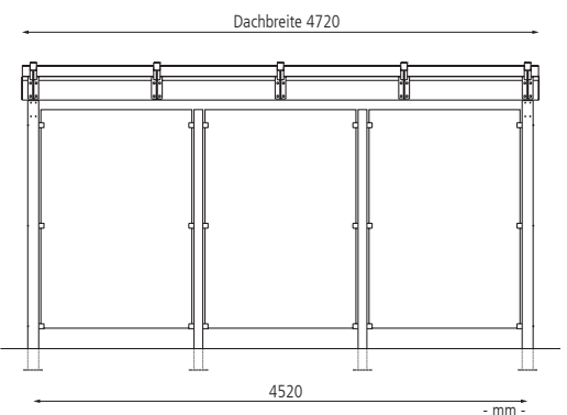
Frontansicht
